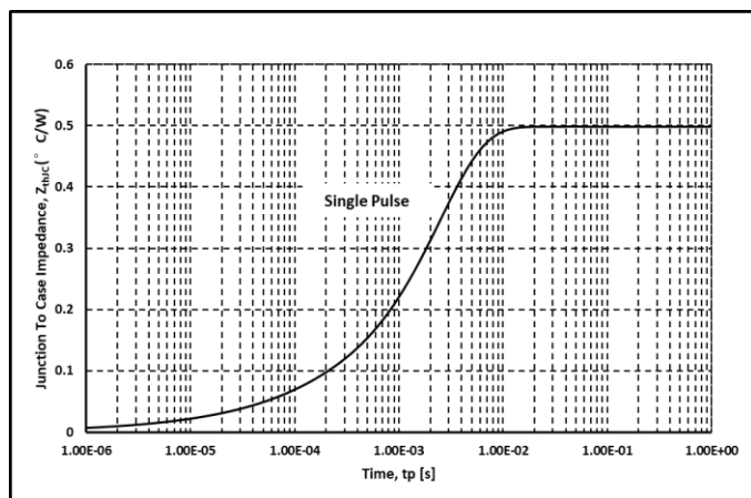
图. 23 热阻曲线
